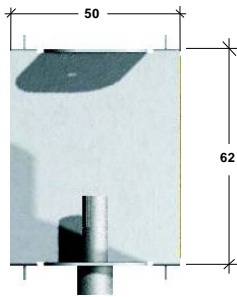
ALZADO
